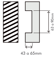
ALVENARIA | VIDRO (Rasgo)
