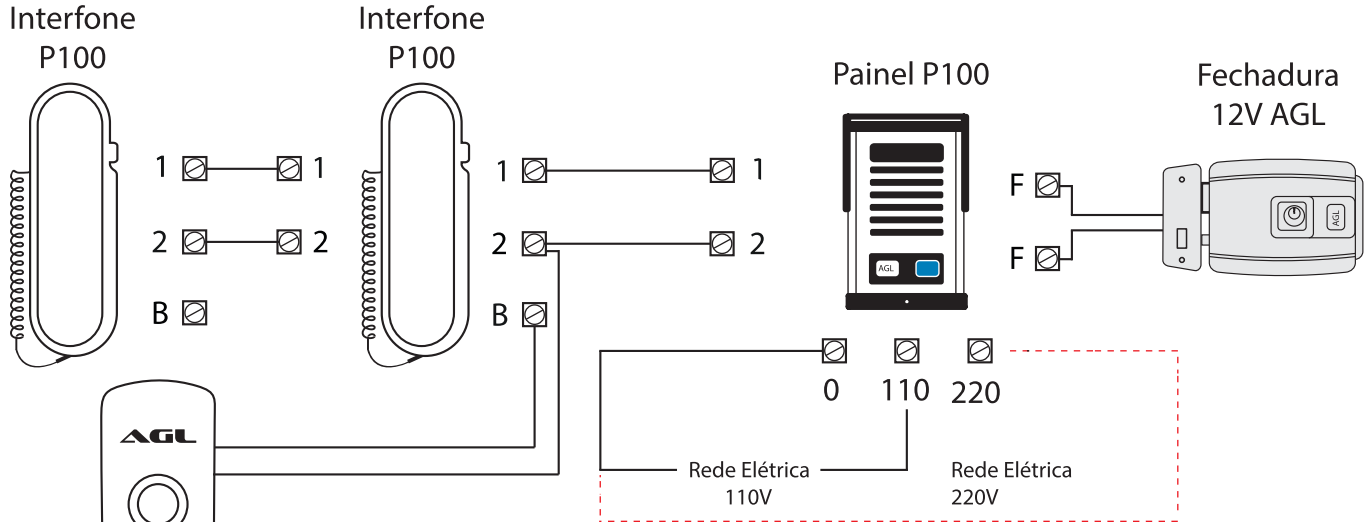
Figura 1 - esquema de ligação com porteiro P100 AGL
