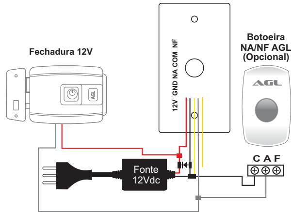
Figura 2 - esquema de ligação com fechadura convencional
