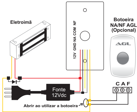
Figura 1 - esquema de ligação com eletroímã/solenóide
